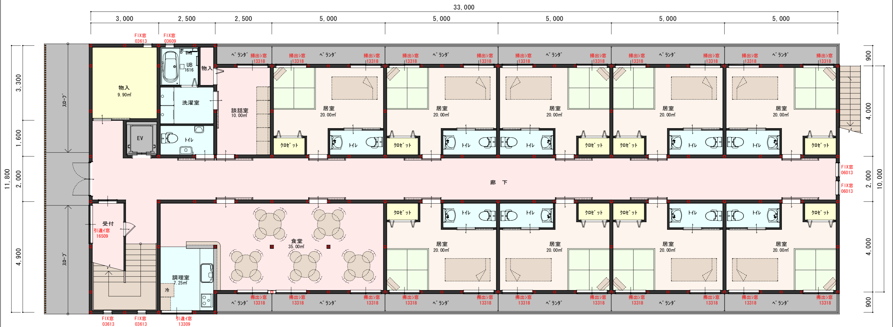
1階平面図 S=1/100
